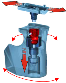
Handgriff ‚CIRCULUS 3D‘ für KK SPORT / WORLDCUP / METALLIC / LADY
